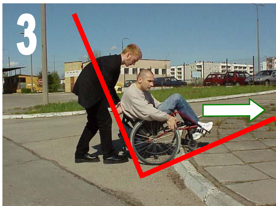
Stawiamy mniejsze kółka pomocnicze na przeszkodzie i jednocześnie pchamy wózek do przodu
